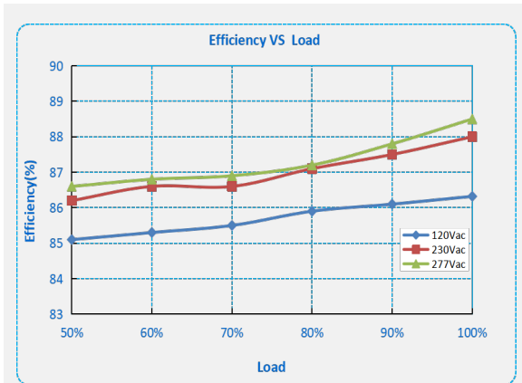
L1-100X-012/024
